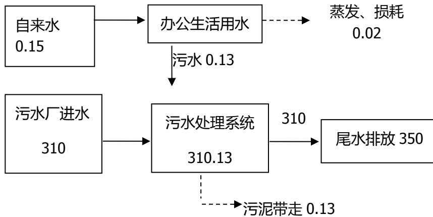
图 2-1 营运期水平衡图 单位：m 3 /d（以监测当天流量计算）
