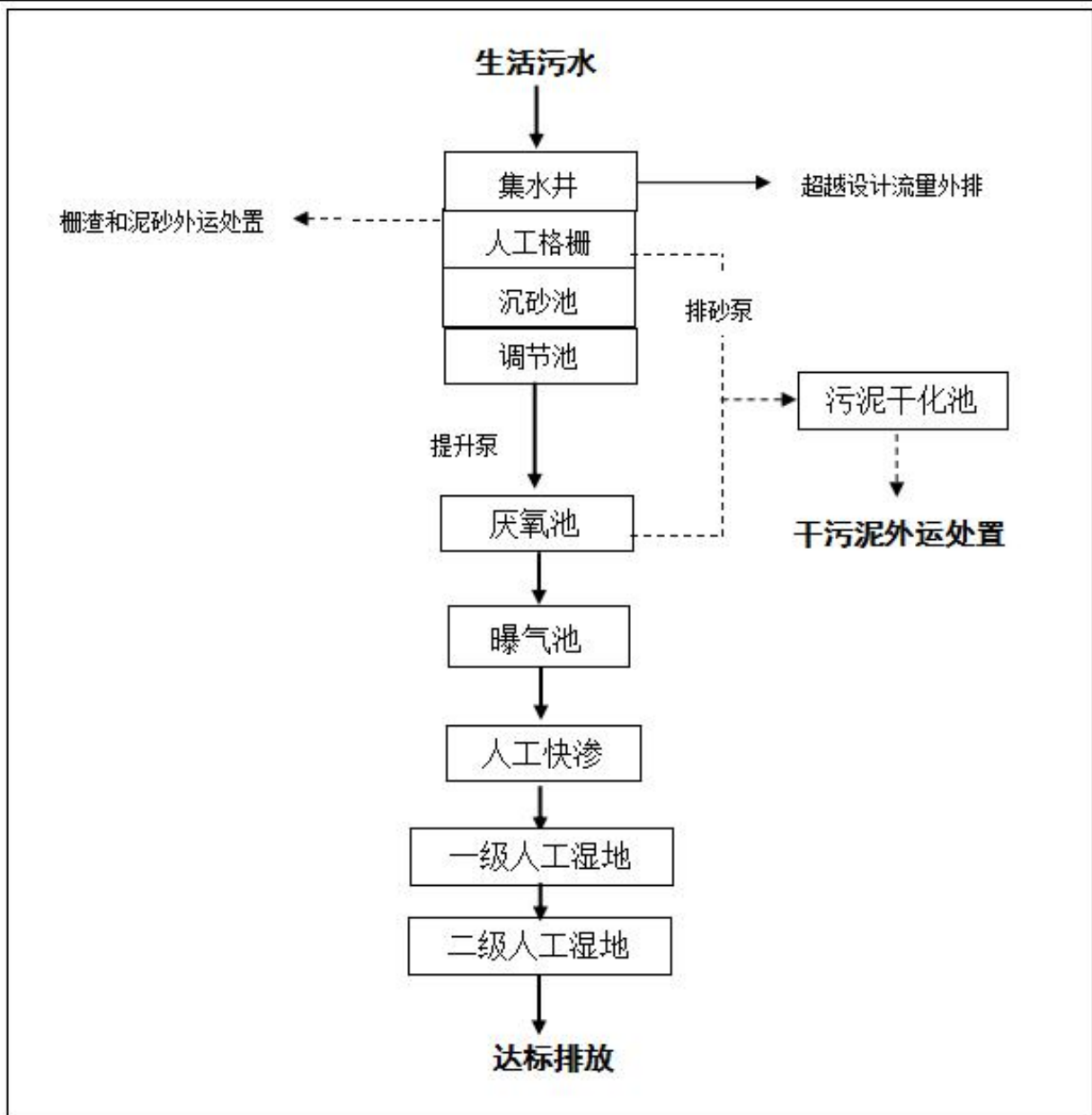
图 2-2 项目工艺流程及产污环节图
