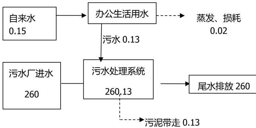
图 2-1 营运期水平衡图 单位：m 3 /d（以监测当天水量计算）
