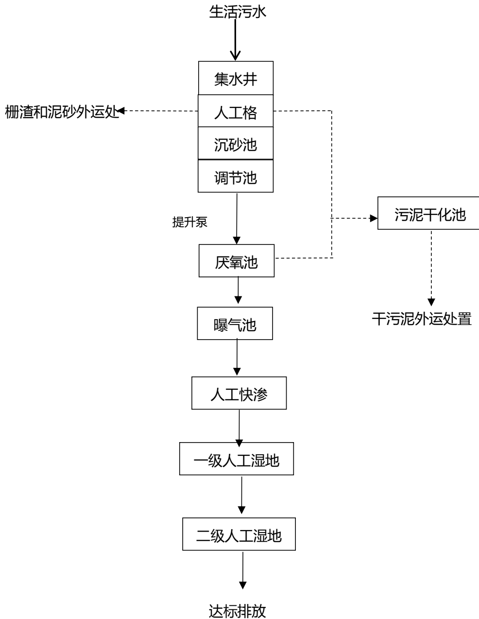
图 2-2 项目生产工艺流程及产污环节图
