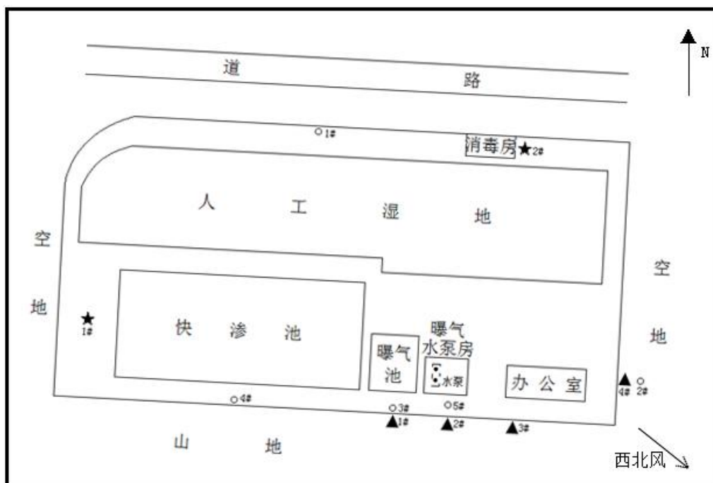
图 6-1 布点示意图 ●: 噪声源 ▲: 其他噪声检测点 ★: 废水检测点 ○: 无组织排放废气检测点
