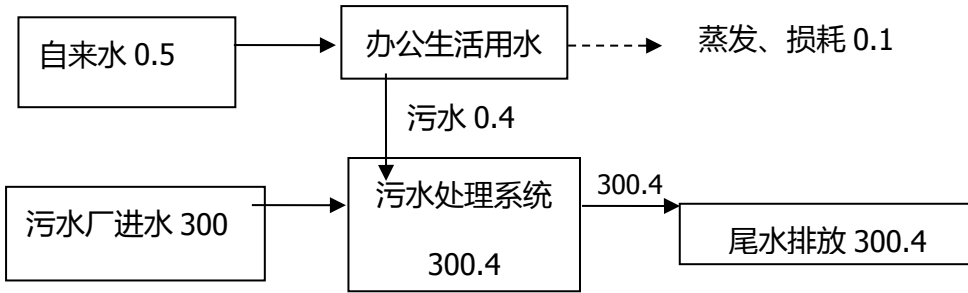
图 2-1 运营期水平衡图 单位： \text{m}^3/\text{d}
