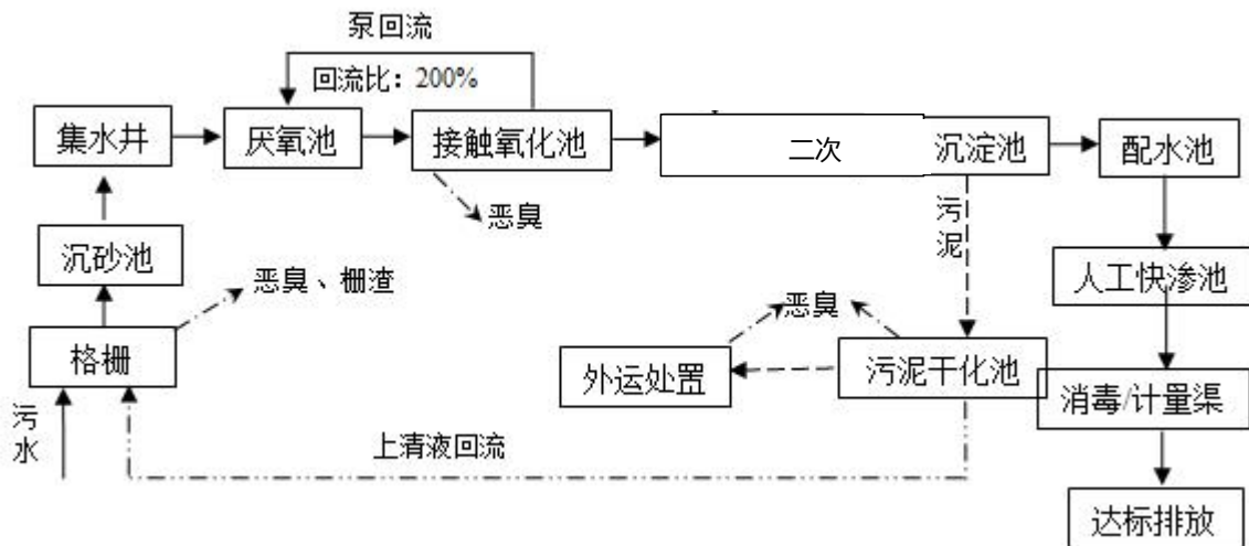
图 2-2 项目生产工艺及产污环节图
