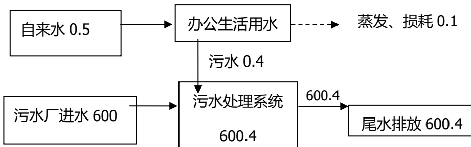
图 2-1 营运期水平衡图 单位: m 3 /d
