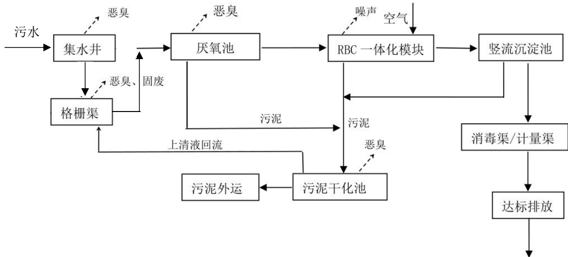
图 2-2 项目生产工艺及产污环节图
