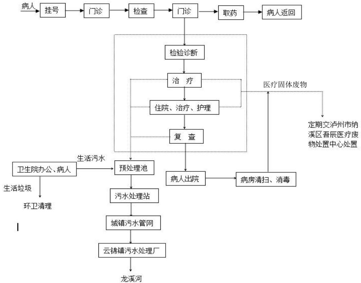
图 2-2 运营期工艺流程图
