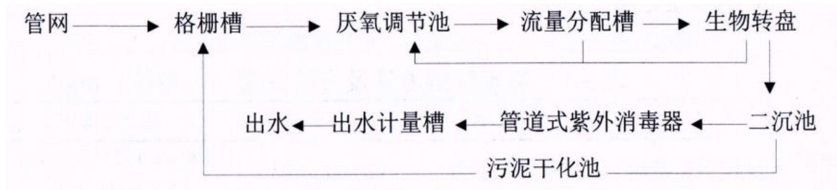
图 2-2 项目生产工艺及产污环节图
