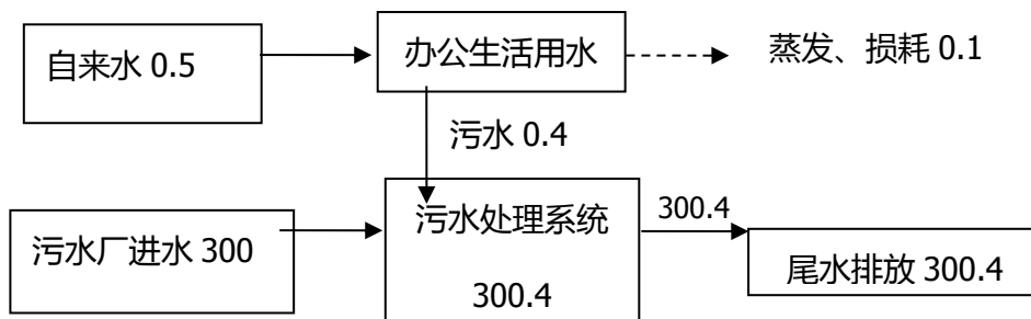
图 2-1 营运期水平衡图 单位：m 3 /d
