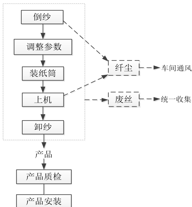
图 3-1 项目营运期工艺流程及产污图
