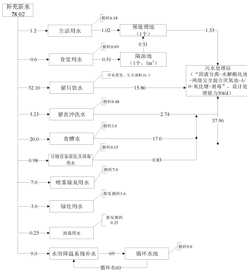
图 2.4-1 全场水平衡图 (单位: m 3 /d)
