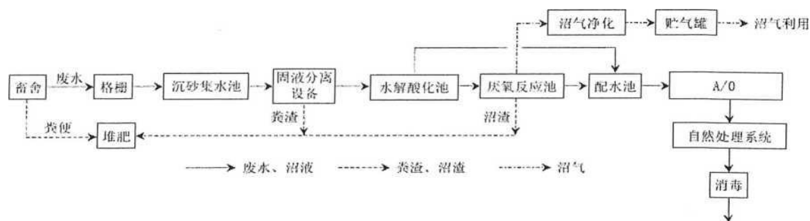
图 2.6-9 污水处理站工艺流程图
