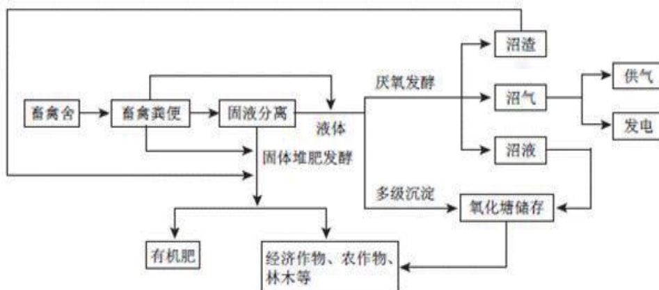
图 2.6-8 农业部推荐种养循环基本工艺流程
