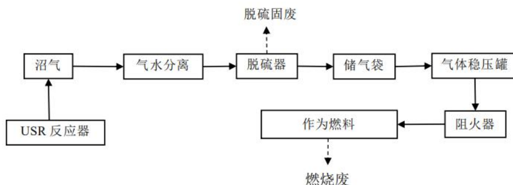
图 2.6-11 沼气净化工艺流程图
