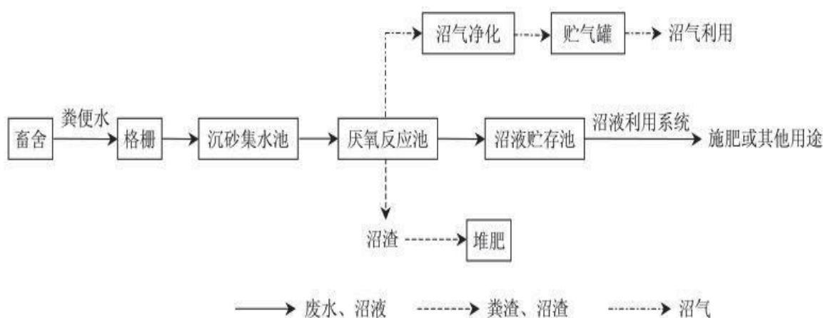
图 2.6-5 模式 I 基本工艺流程
