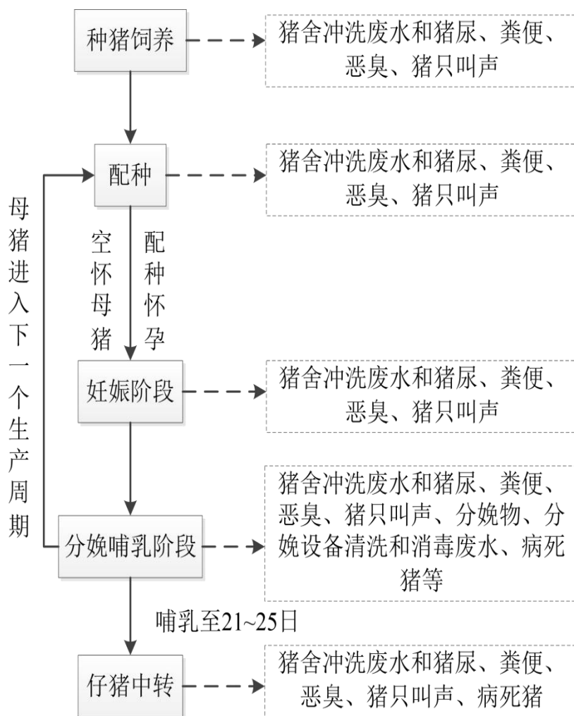
图 2.6-3 养殖工艺流程及产污位置示意图
