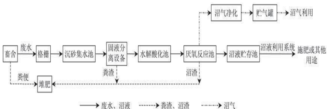
图 2.6-6 模式 II 基本工艺流程
