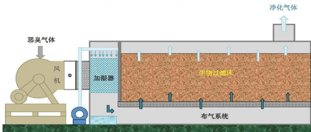
生物过滤法除臭工艺流程示意图
