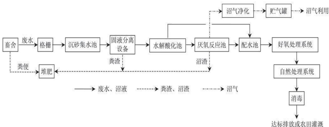
图 2.6-7 模式 III 基本工艺流程
