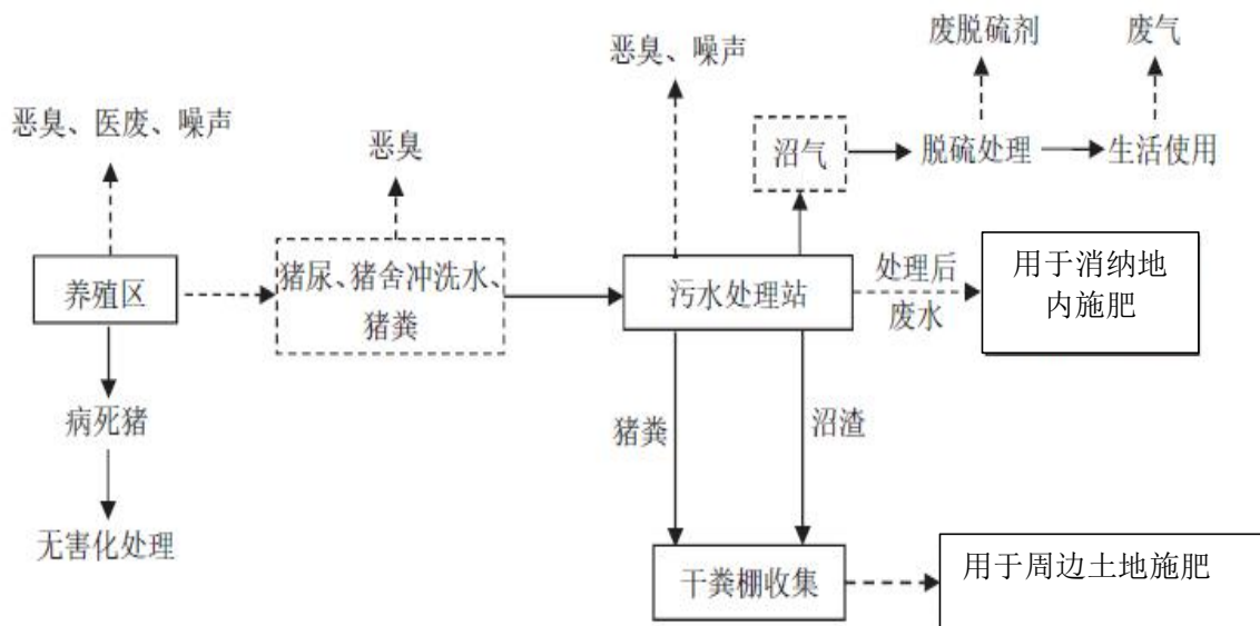
图 2.6-4 营运期工艺流程及产污位置示意图
