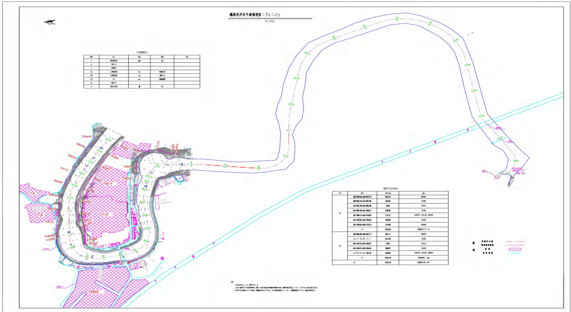
附图三 项目平面布置图
